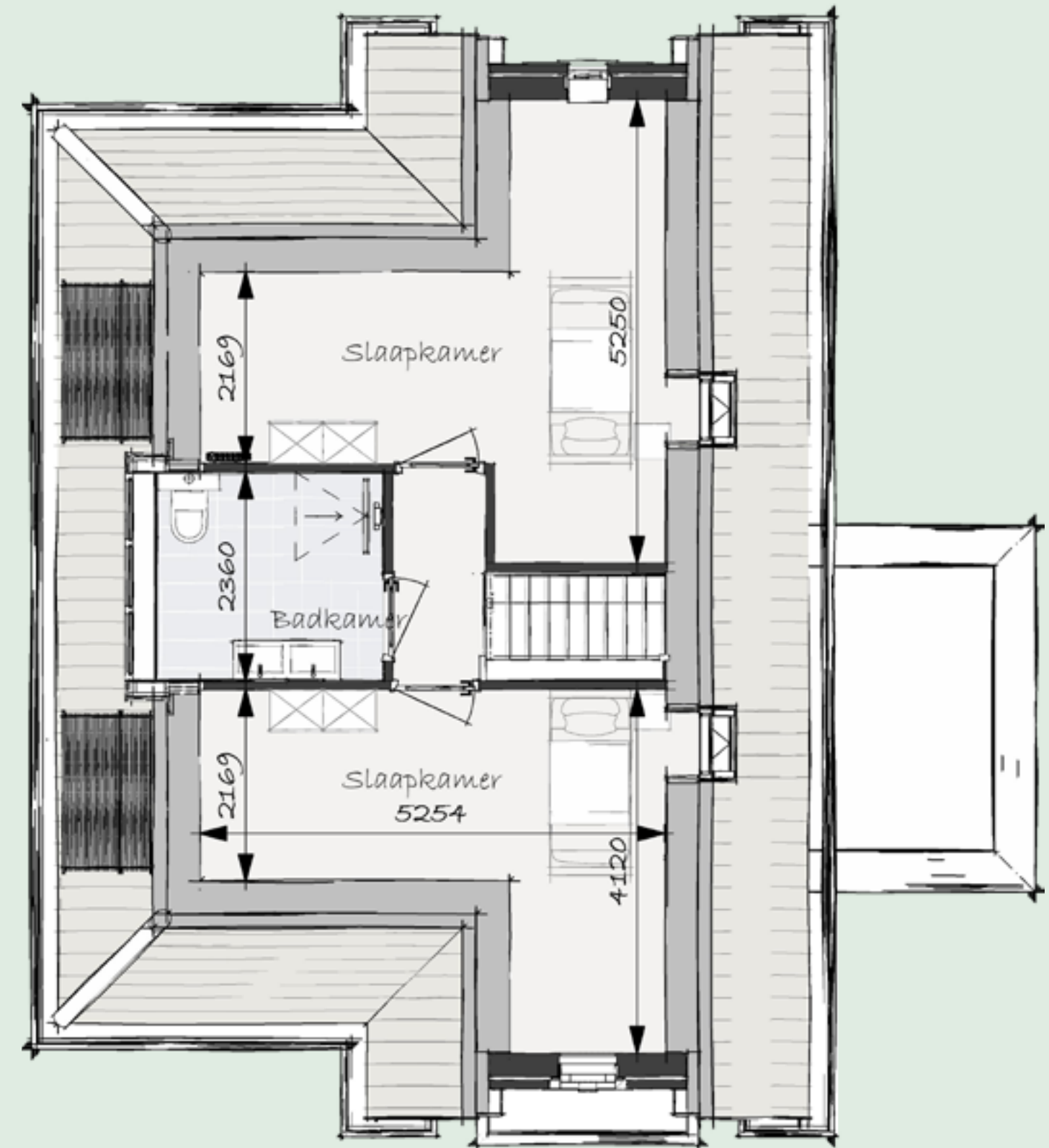
2e Verdieping
